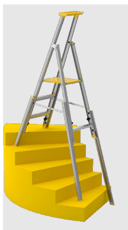
Ajuste de altura individualizado para cada perna
