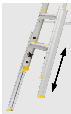
Detalhes do sistema de fixação
