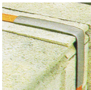
Ref. 87 - 25/35/50 Tubo protetor em PVC para cintas com 25/35 ou 50 mm de largura. Para amarração de cargas abrasivas
